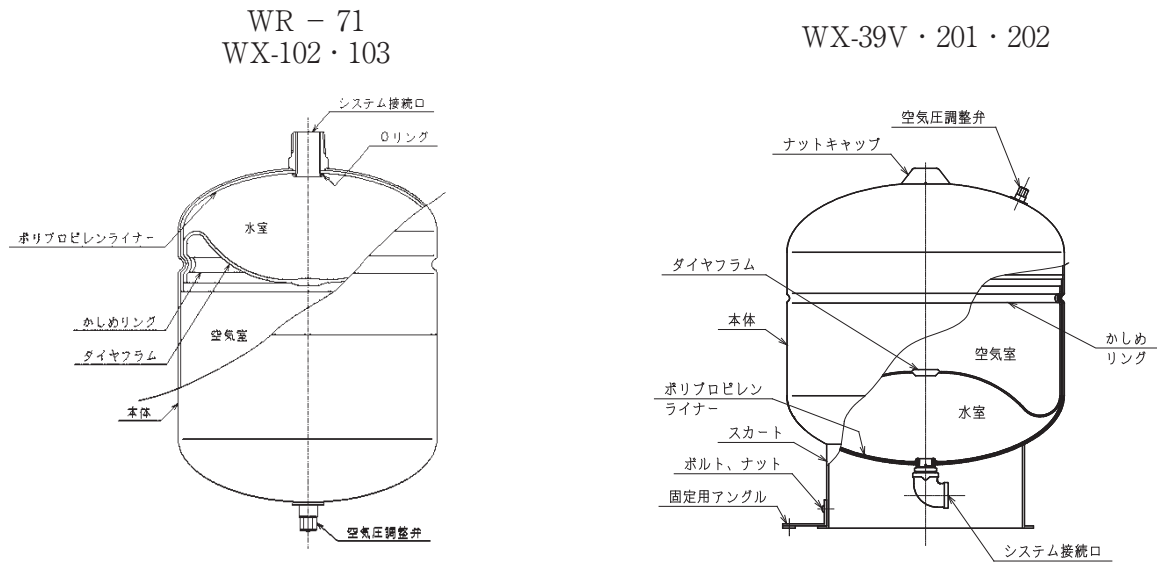
図1-1 タンク構造図
